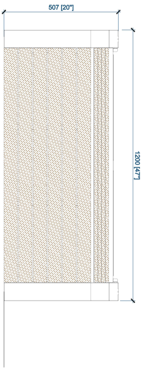
PLAN PLANTA
