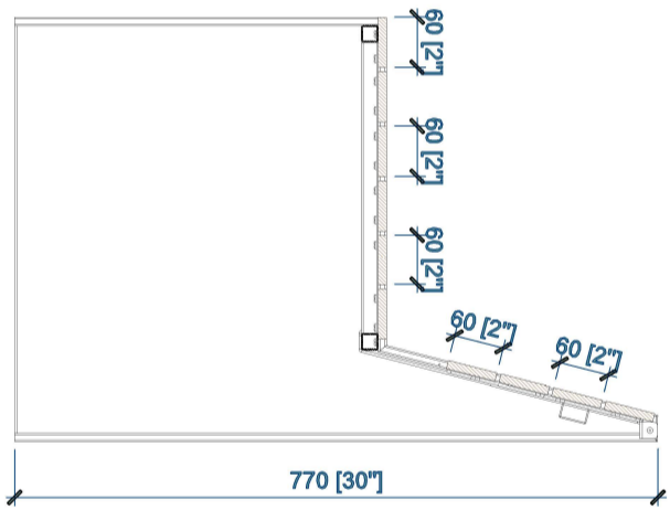
SECTION AA SECCIÓN AA
